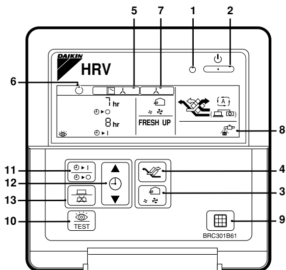
BRC301B61: Τηλεχειριστήριο για VRV
