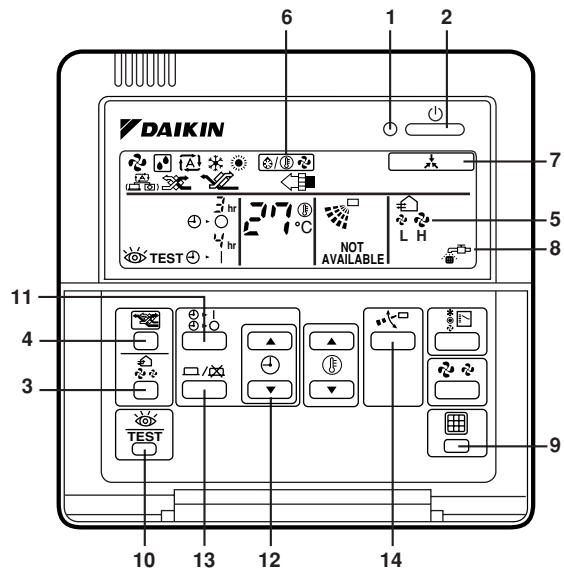
BRC1C51, 61, 517: Τηλεχειριστήριο για VRV
