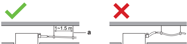
a Ράβδος ανάρτησης ✓ Επιτρέπεται ✗ Δεν επιτρέπεται
