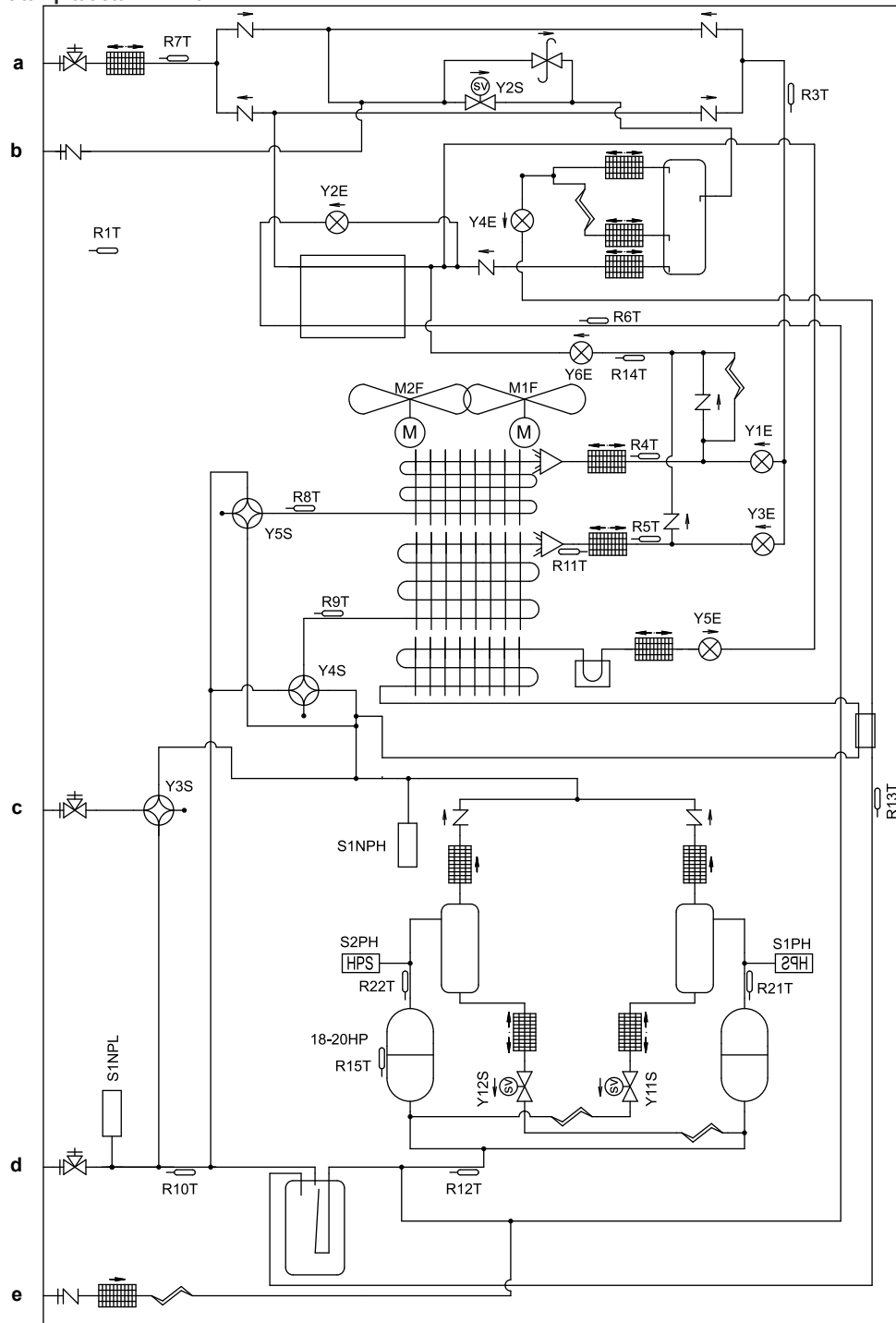
Διάγραμμα σωληνώσεων: 14~20 HP
