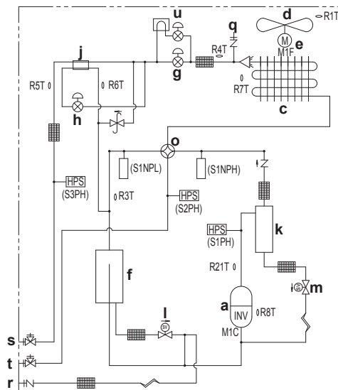
Διάγραμμα σωληνώσεων: RXYQQ14~20
