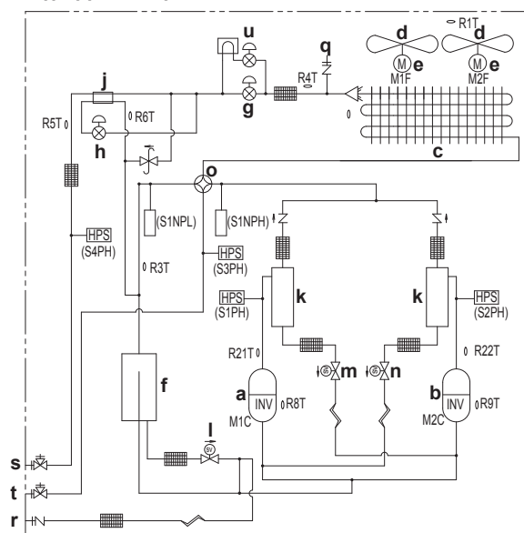
Διάγραμμα σωληνώσεων: RXYQQ14~20
