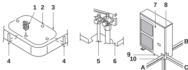
Εικόνα - Αγωγοί εξωτερικού χώρου σε τέσσερις κατευθύνσεις
