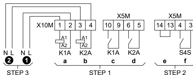
STEP 1 Εγκατάσταση κιτ ρελέ έξυπνου δικτύου
