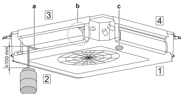
a Πλαστικό δοχείο νερού με μήκος σωλήνα \geq 100 mm b Θέση αντλίας αποχέτευσης και φλοτέρ c Έξοδος εκκένωσης για συντήρηση (με ελαστική τάπα). Χρησιμοποιήστε αυτή την έξοδο για να αποστραγγίσετε νερό από τη λεκάνη εκκένωσης.
