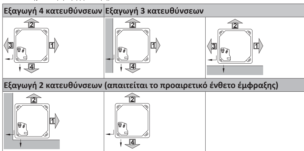
16-1 Σχέδιο εξαγωγής (κάτοψη)
