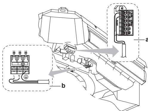
a Κλέμα τηλεχειριστηρίου b Κλέμα παροχής ρεύματος
